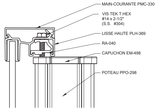
DÉTAIL A VUE 1:2
